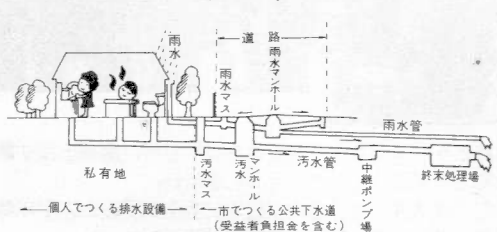
公共下水道のしくみ(分流式)
